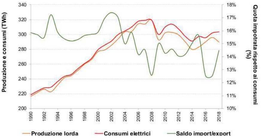
Figura 5.6: Andamento della produzione e del consumo di energia elettrica e quota importata rispetto ai consumi
