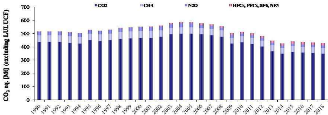
Figura 4.7: Emissioni nazionali di gas serra dal 1990 al 2018, escluso foreste e suolo (Mt CO 2 eq) Fonte: ISPRA
