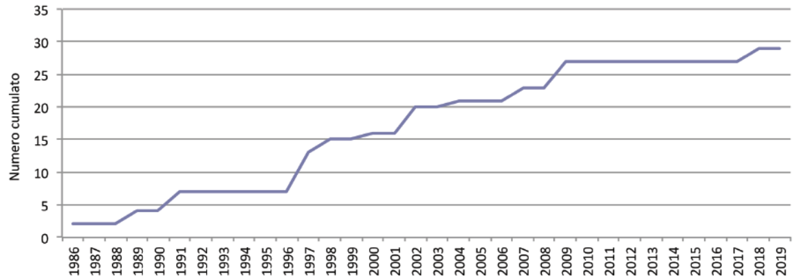
Figura 1.17: Variazione annuale del numero cumulado delle 29 Aree Marine Protette
