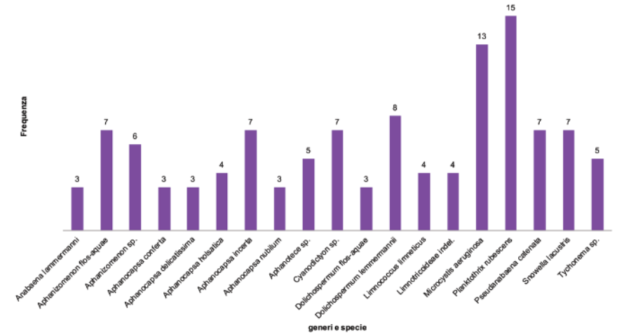
Figura 10.5: Frequenza dei generi e delle specie più ricorrenti in 21 laghi considerati (2018)
