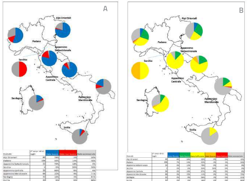
Figura 2.5: Stato chimico (A) ed ecologico (B) dei laghi
