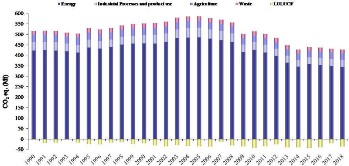
Figura 4.8: Emissioni e assorbimenti di gas serra dal 1990 al 2018 per settore (Mt CO 2 eq.) Fonte: ISPRA
